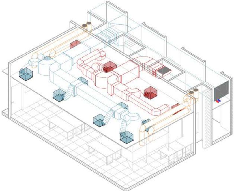
Laboratorio tipo - Impianti meccanici Tipologico distribuzione secondaria
